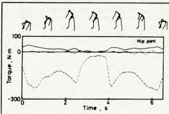
Figuren viser belastninga på hoftedeledet hos en robot under en løfte-operasjon som tar seks sekund.
